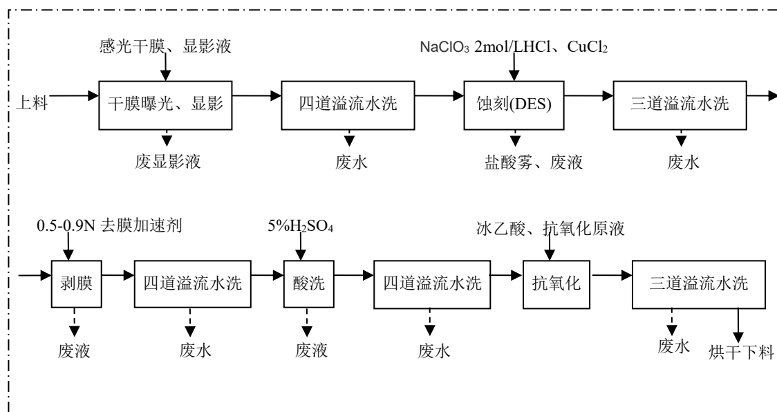
图 3-2 蚀刻环节工艺流程及产污环节
