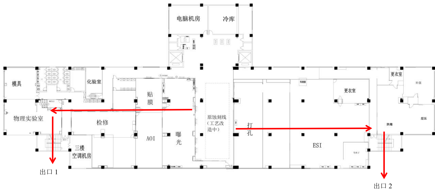
三楼平面布置图
