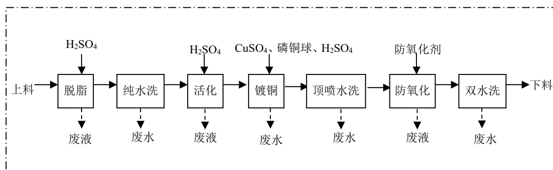
图 3-4 精密镀铜环节工艺流程及产污环节
