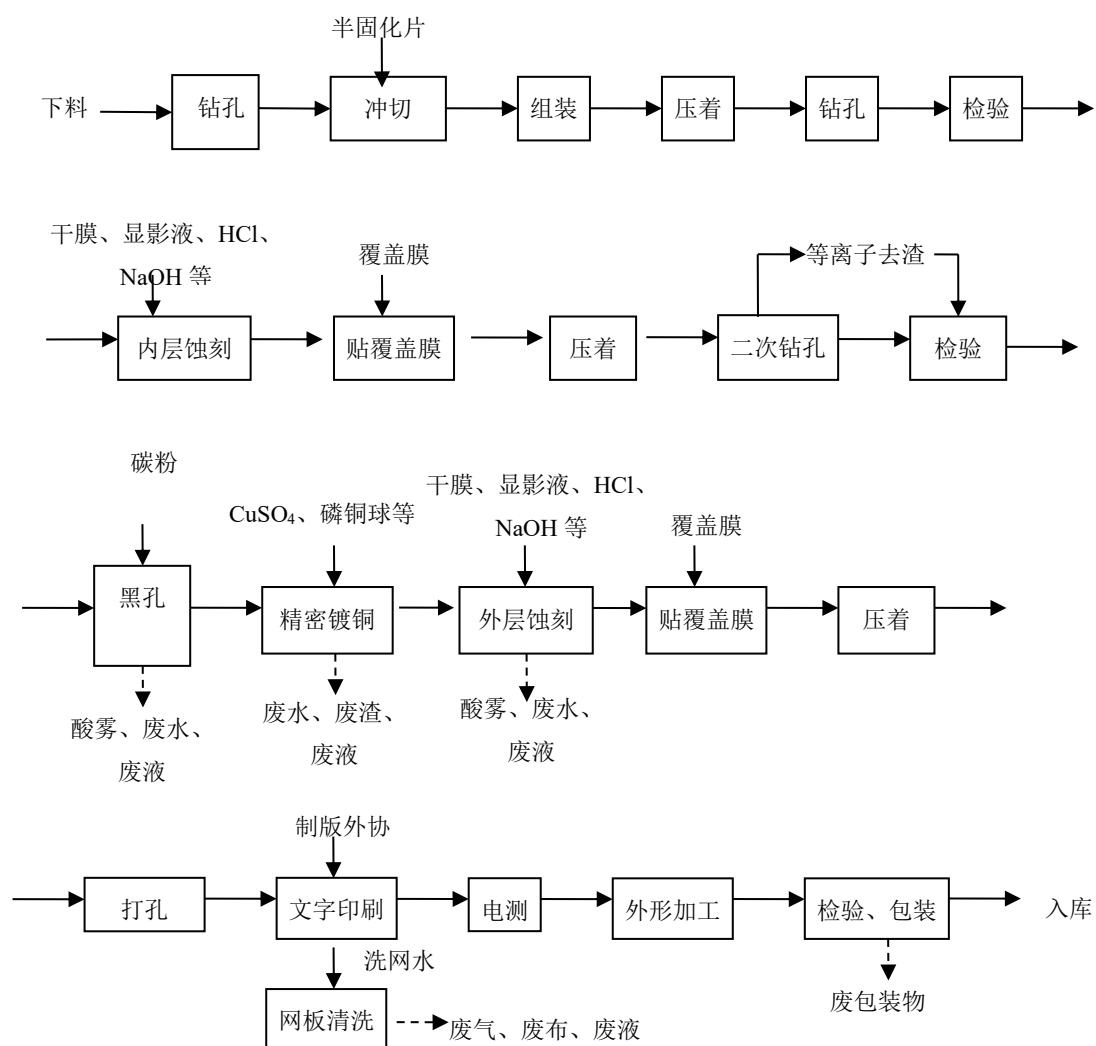
图 3-1 翔岳厂印制绕性线路板总体流程图
