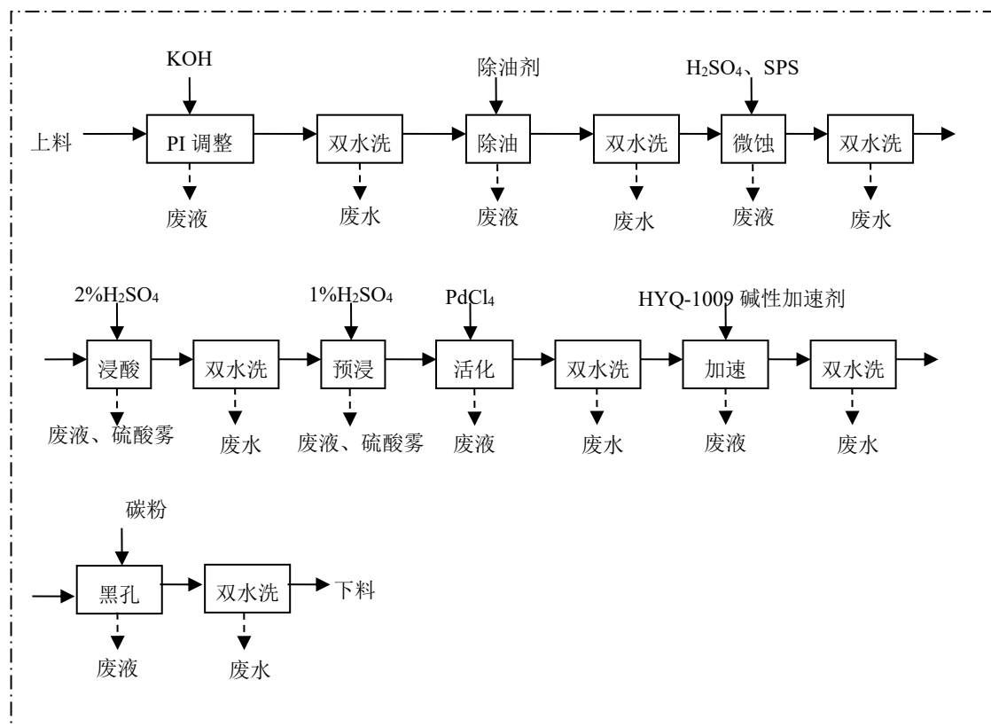
图 3-3 PTH (黑孔) 环节工艺流程及产污环节
